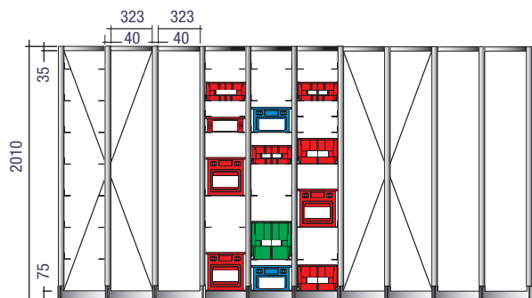
profondità scaffalatura 500 mm
