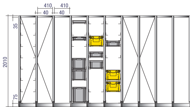
profondità scaffalatura 600 mm
