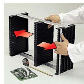
spostamento del divisorio centrale
