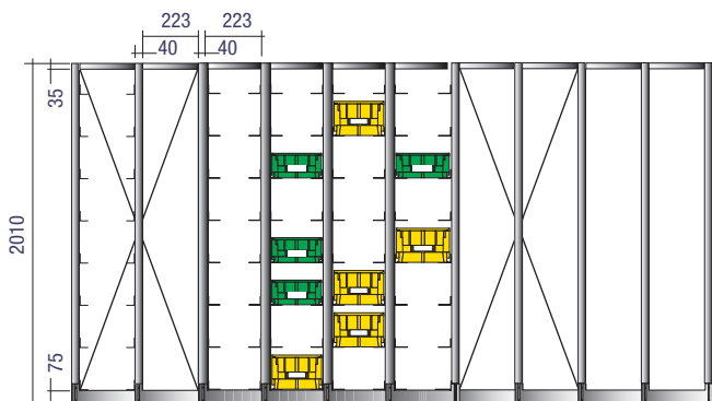
profondità scaffalatura 350 mm
