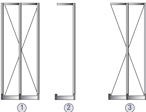
profondità scaffalatura 600 mm
