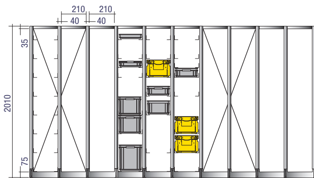
profondità scaffalatura 300 mm
