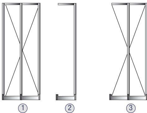
profondità scaffalatura 300 mm
